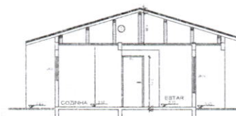
CORTE BB
