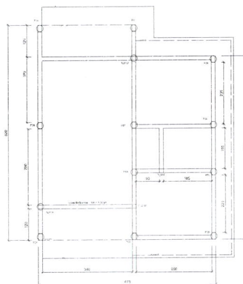
ESQUEMATICO BALDRAMES E VIGAS SUPERIORES
