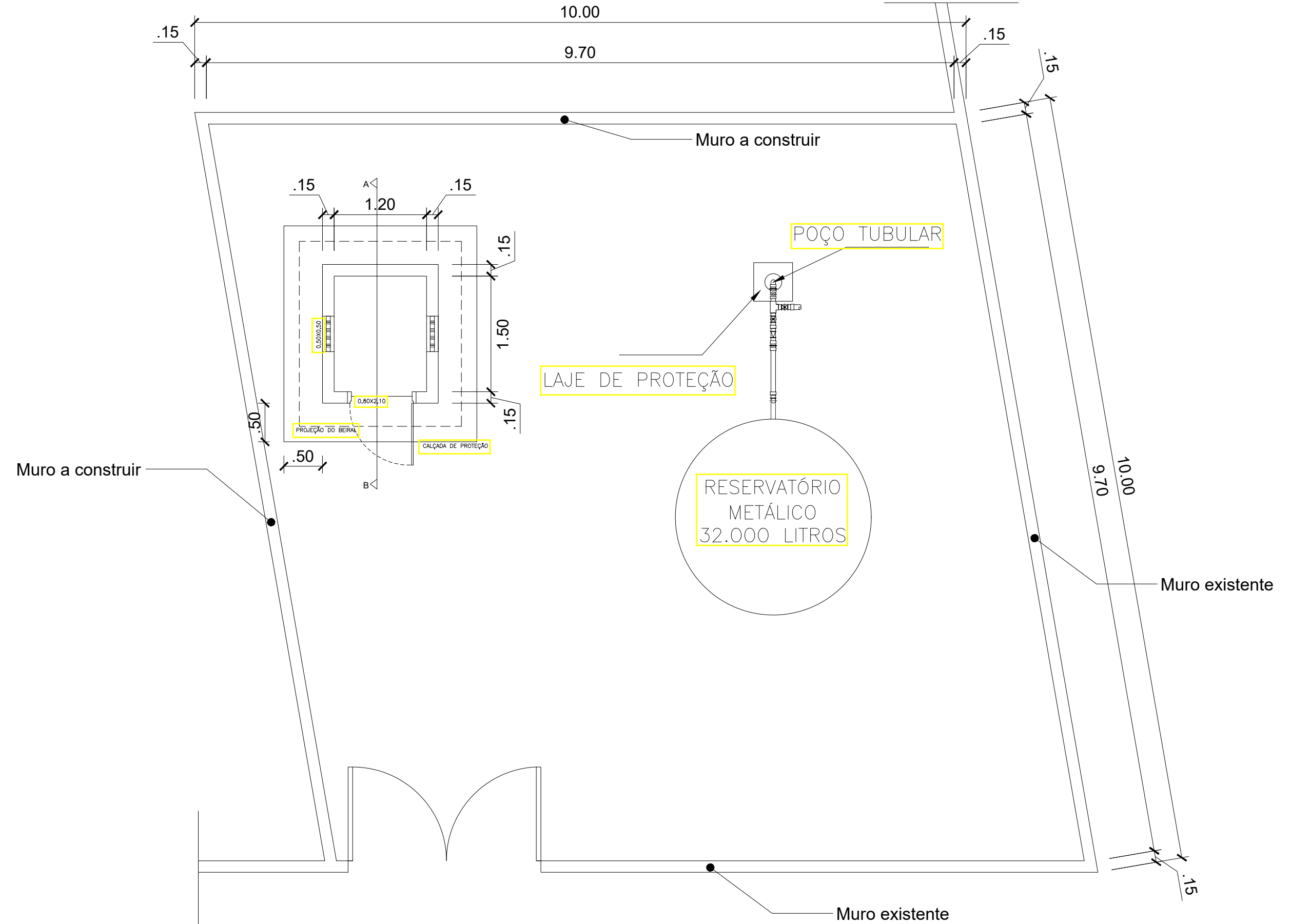
PLANTA BAIXA ESC: 1/50
