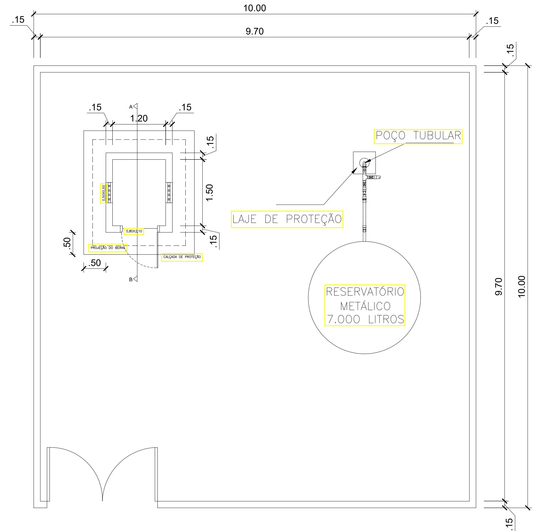
PLANTA BAIXA ESC: 1/50
