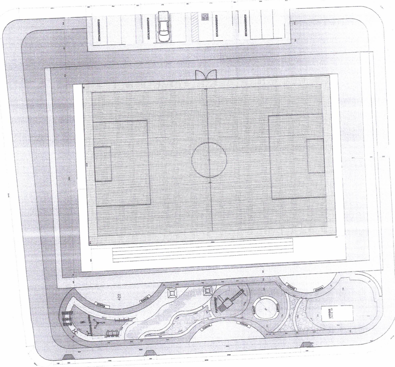
PLANTA DE LAYOUT E PISO ESC. 1:1000
