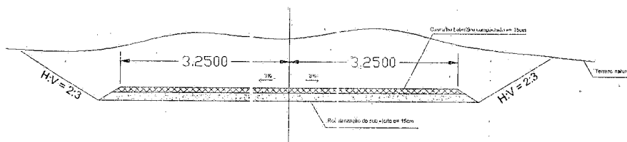
SEÇÃO TRANSVERSAL EM CORTE
