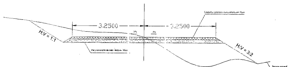
SEÇÃO TRANSVERSAL TIPO MISTA
