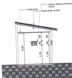
1 CORTE TRANSVERSAL - Vestiários ESCALA 1/50
