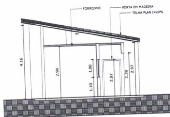
1 CORTE TRANSVERSAL - SALAS DE AULA ESCALA 1/50
