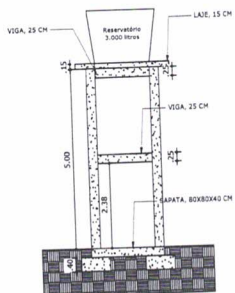
1 CORTE ESTRUTURA PARA RESERVATÓRIO ESCALA 1/50
