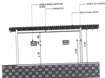
1 CORTE LONGITUDINAL - Vestiário masculino ESCALA 1/50
