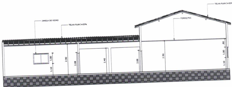
1 CORTE LONGITUDINAL - SALAS DE AULA ESCALA 1/50
