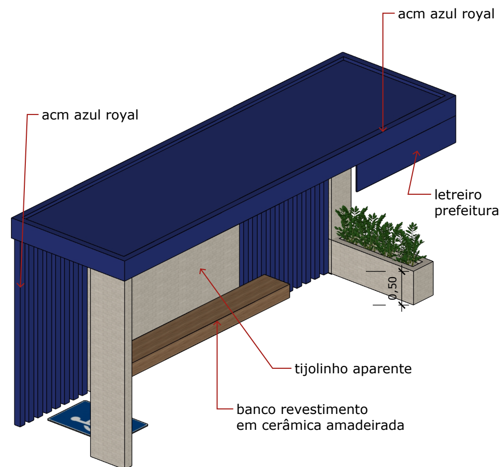
05 perspectiva escala 1:50
