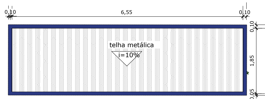
02 cobertura escala 1:50
