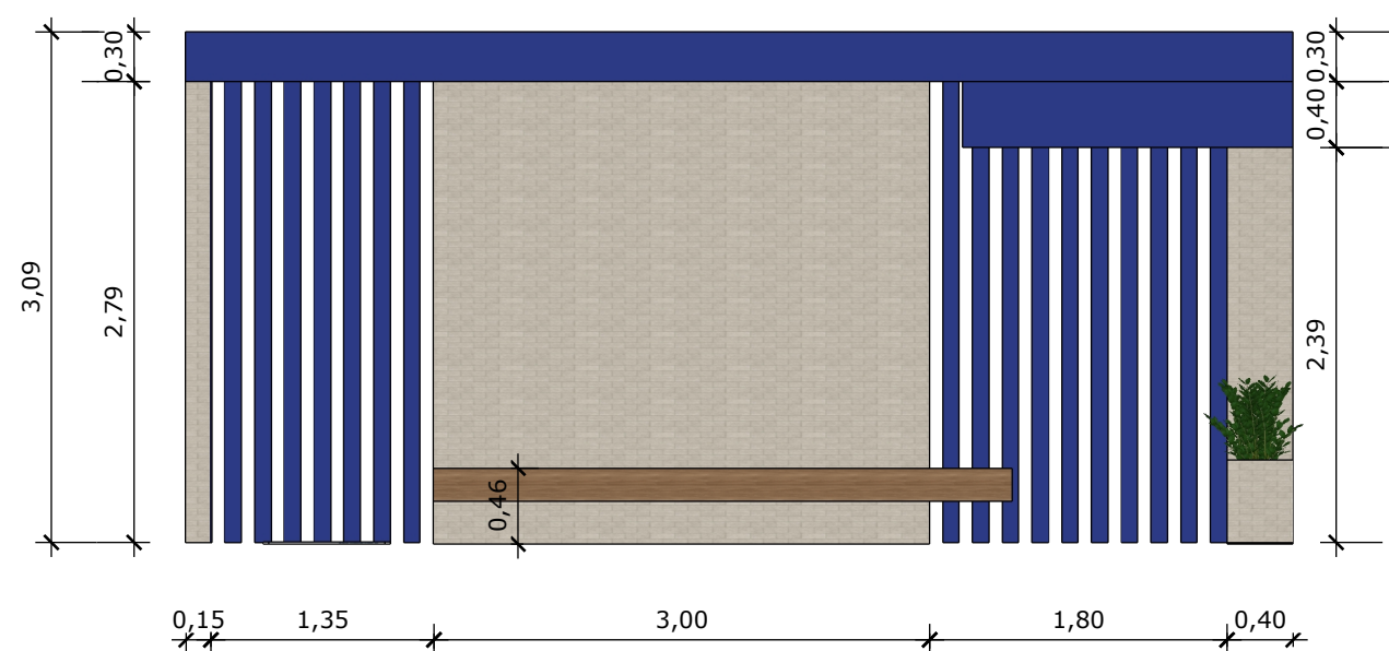
03 vista frontal escala 1:50
