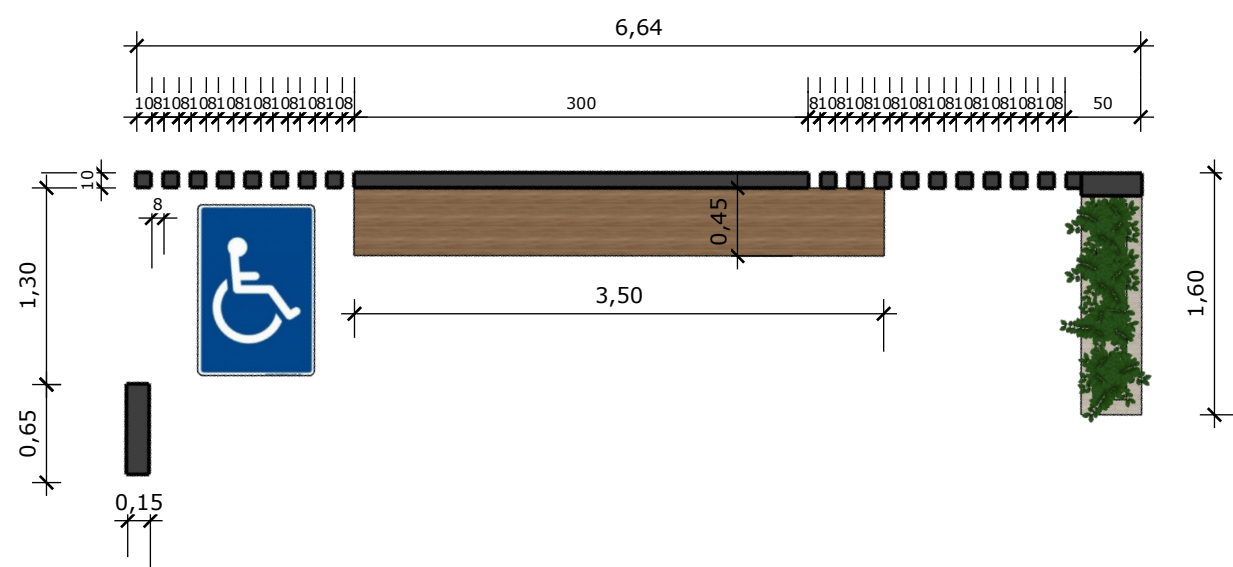
01 vista superior escala 1:50
