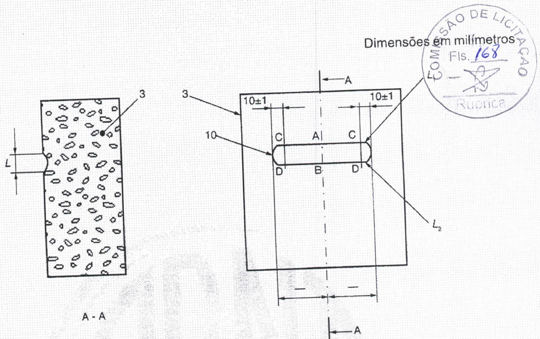
Figura C.2 — Medição da cavidade na amostra ensaiada
